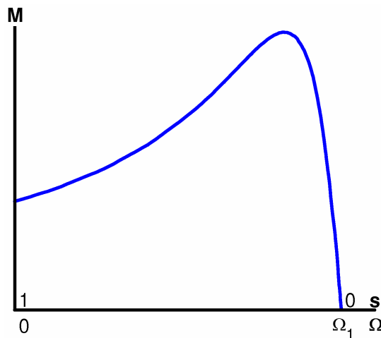
Fig. 1: Par de un motor asíncrono
