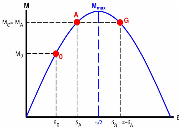
Fig. 5: La máquina perderá estabilidad si durante las oscilaciones el ángulo de par supera el valor \delta_G .
