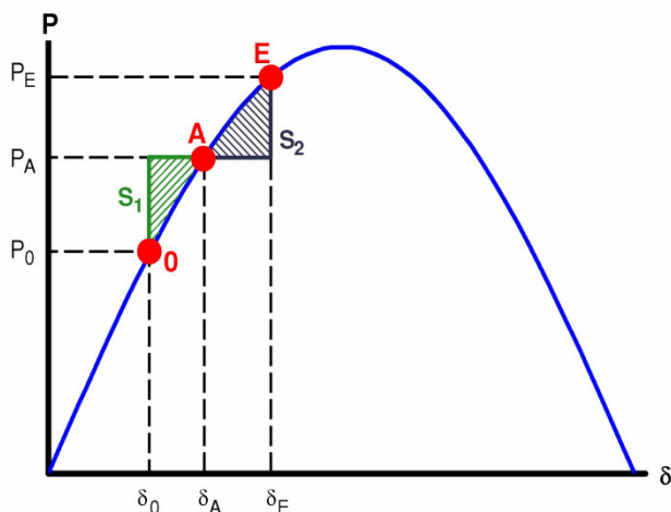
Fig. 6: Método de igualdad de las áreas
