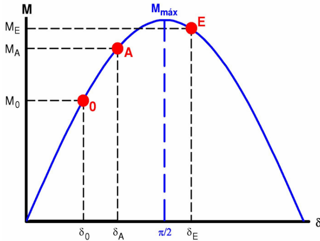
Fig. 4: Funcionamiento estable con \delta_E > \pi/2
