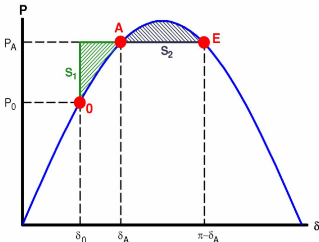
Fig. 7: Límite de estabilidad dinámica
